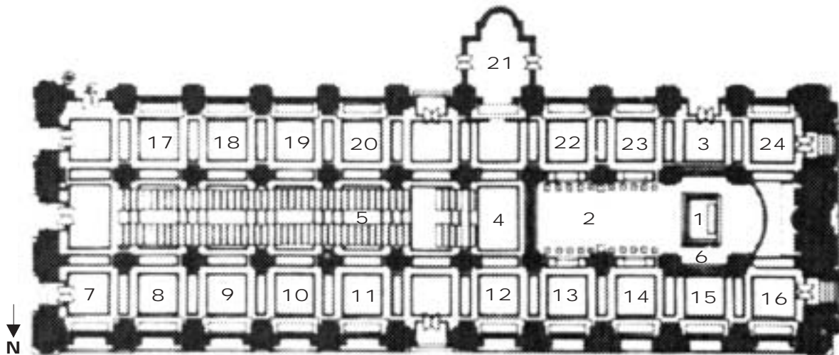
Planta de la Iglesia Catedral de Santiago.
